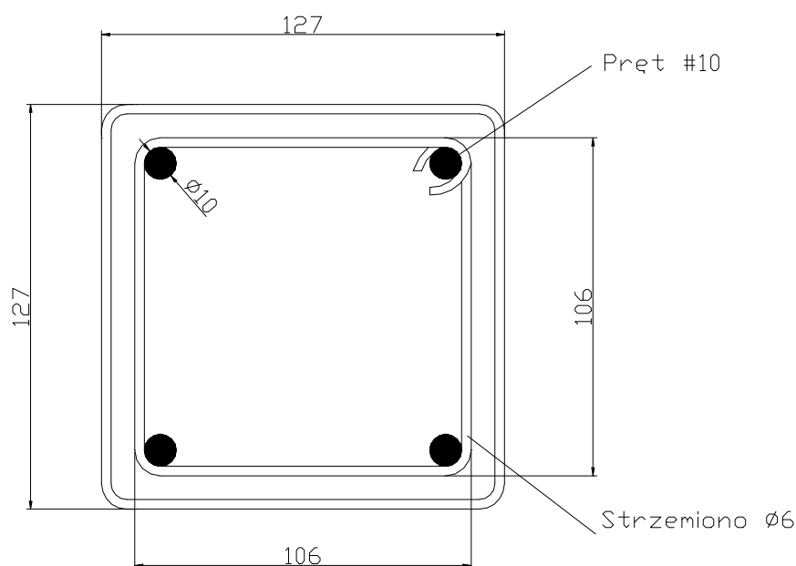
Rys. 9 Zbrojenie słupków w gruncie
